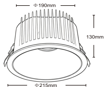
60-65W
